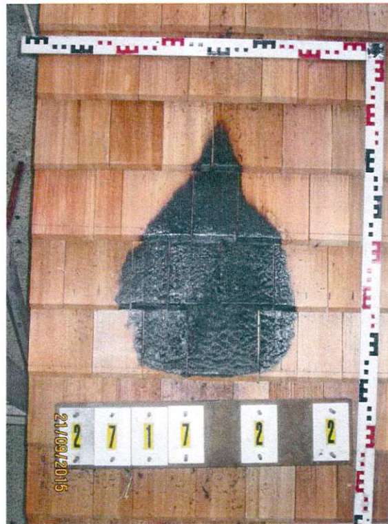
Probedach #6 nach der Brandprüfung Roof sample #6 after flammability test
